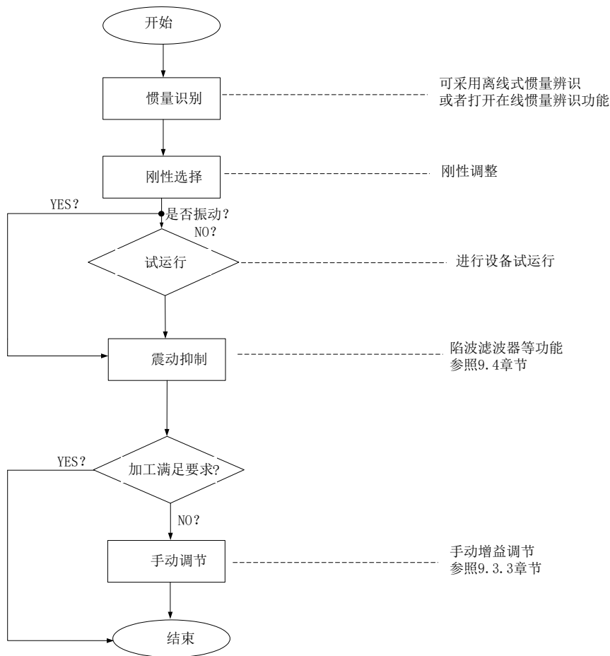
图 9.1.1 增益调节流程图
